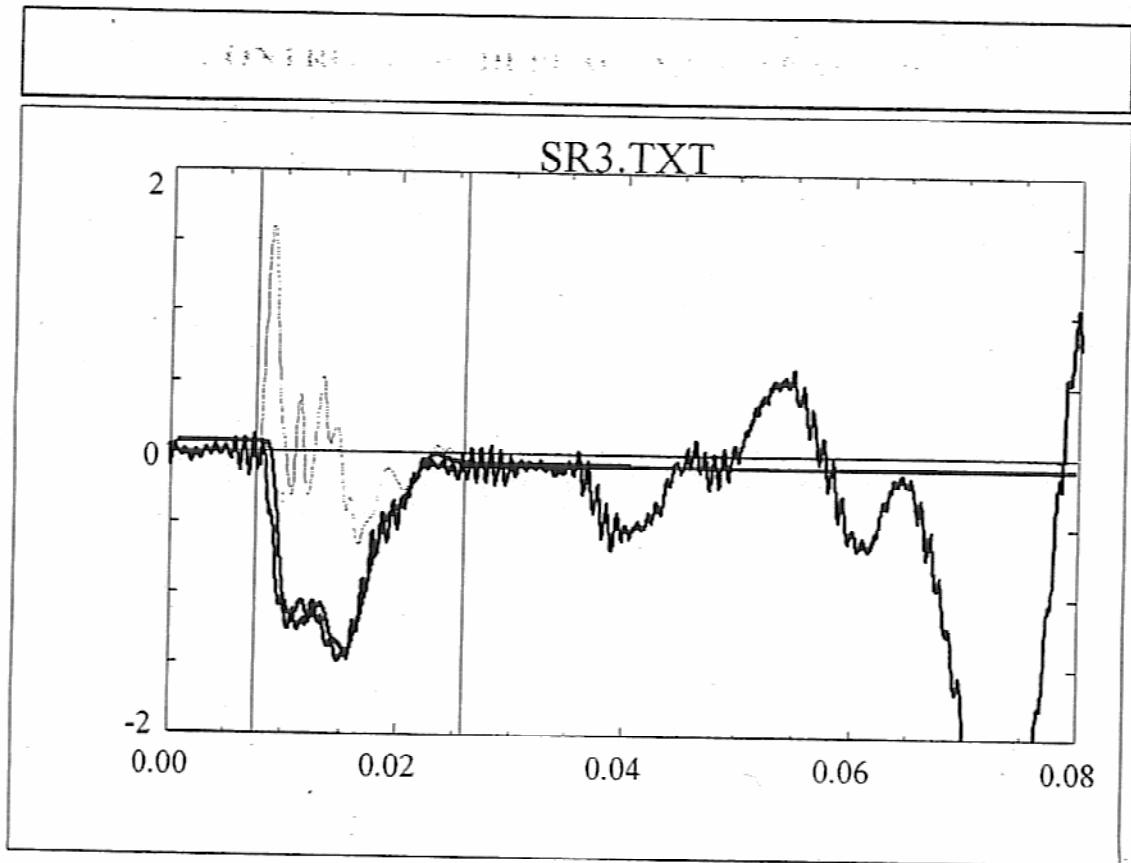
Projet FOREVER : essai de chargement dynamique
